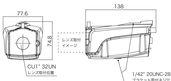
外形図(mm)
