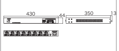
外形図(mm)
