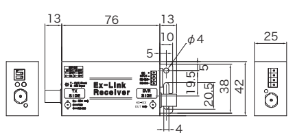
外形図(mm)
