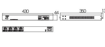
外形図(mm)
